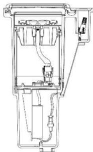
FIGURA 5. Luminaria de acentuación Mérida
