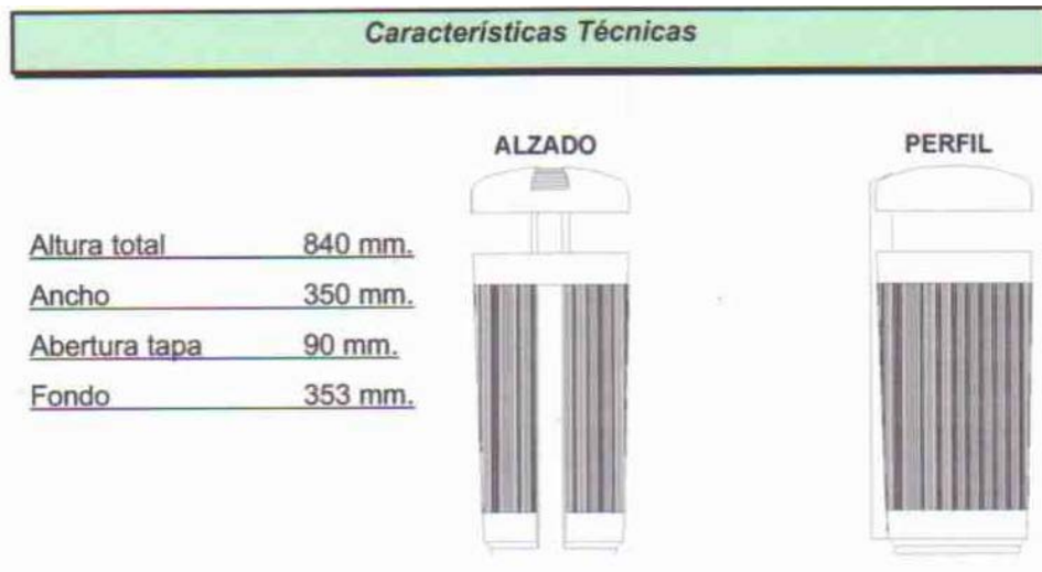
FIGURA 10. Dimensiones de recipientes
